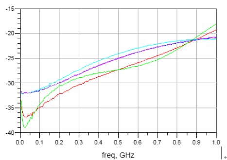
隔离度 Isolation
