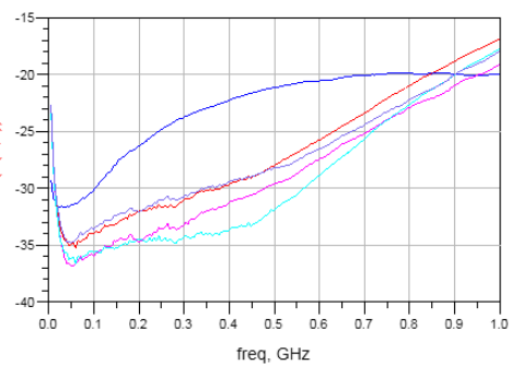
隔离度 Isolation
